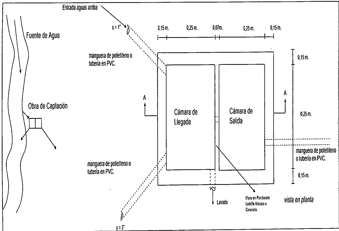
Vista Planta
