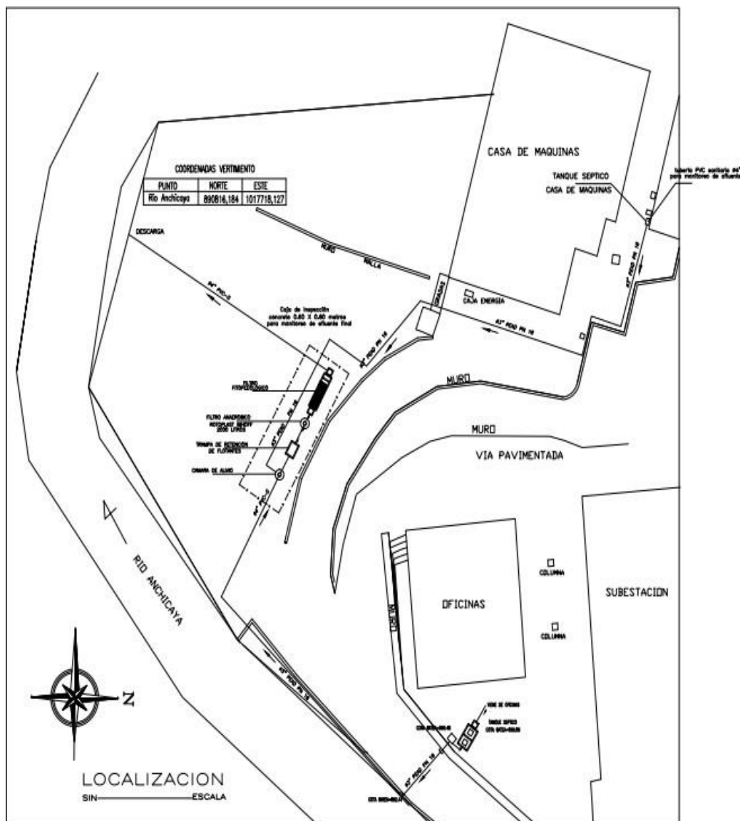
Figura 1. Diagrama del Sistema de Tratamiento. Fuente: Celsia Colombia S.A. E.S.P.-
