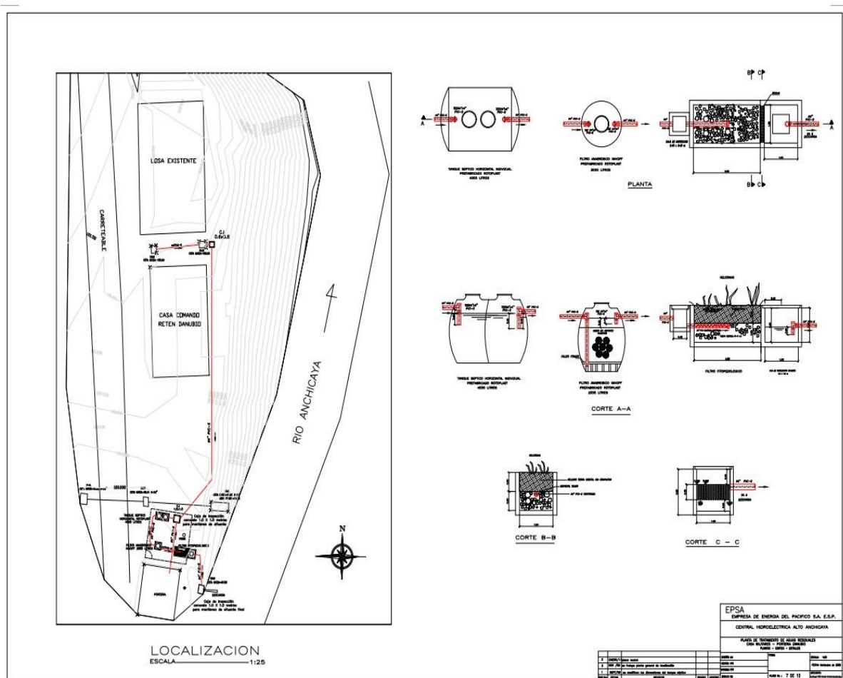
Figura 1. Diagrama del Sistema de Tratamiento. Fuente: Celsia Colombia S.A. E.S.P-
