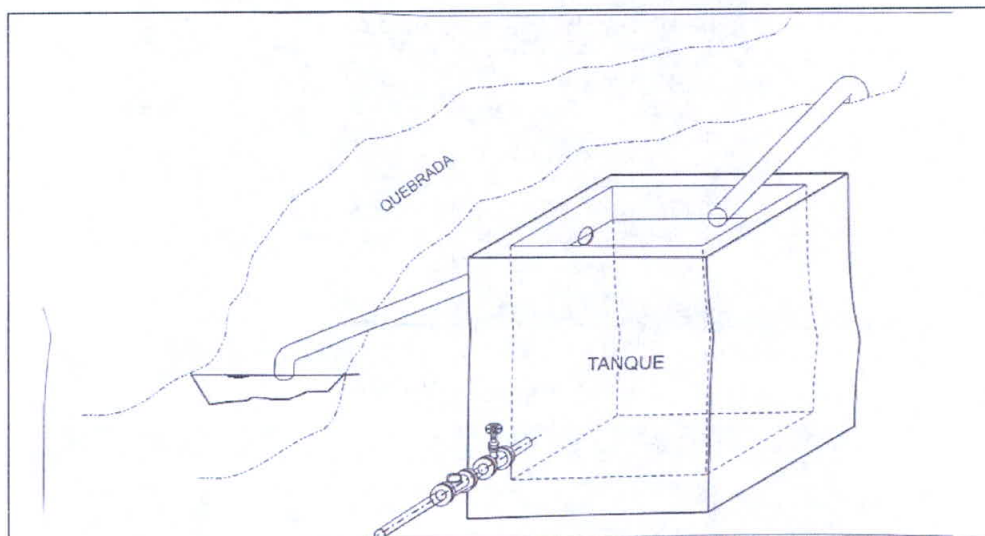
Ilustración 1. Diseños del sistema de captación Campamento Diamante
